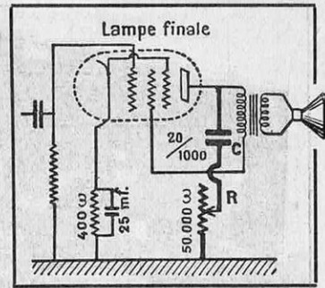
FIG. 15. — CONTROLE DE LA TONALITÉ
