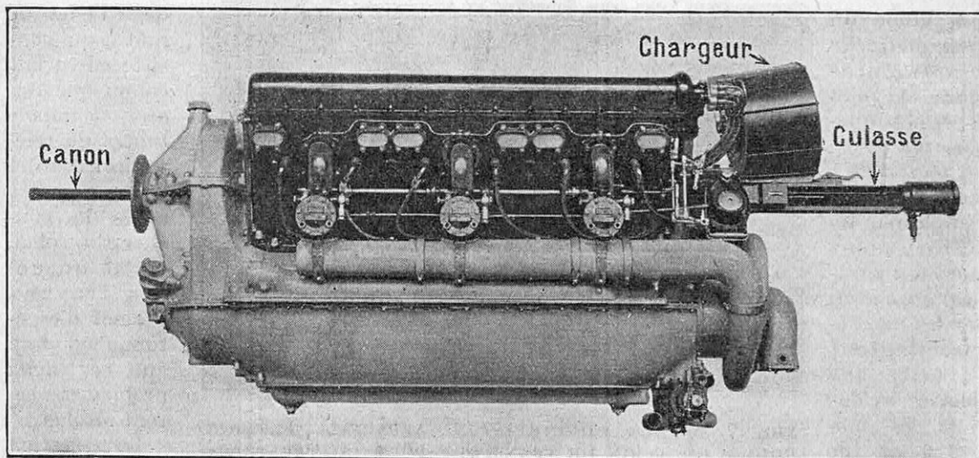
FIG. 8. — MOTEUR-CANON « HISPANO », DE 860 CH (12 Y-C. R. S.)
