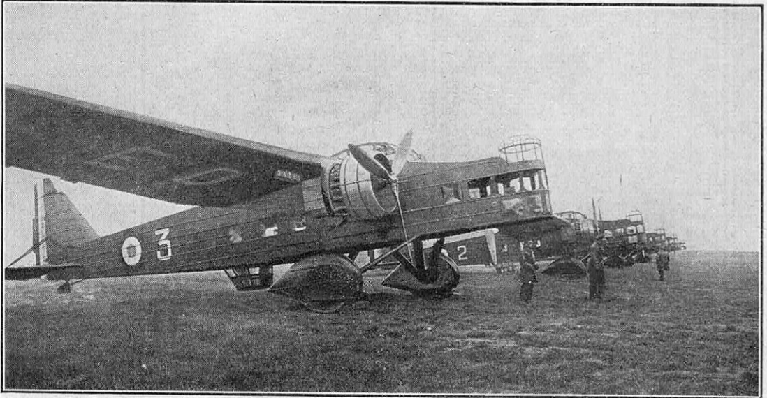
FIG. 2. — ENCORE UN TYPE DE MULTIPLACE DE COMBAT ET DE BOMBARDEMENT : LE « MARCEL-BLOCH-220 ». CET APPAREIL PORTE 1.000 KILOGRAMMES A 1.000 KILOMÈTRES. LA VITESSE ATTEINT, DIT-ON, 290-300 KM-HEURE. LE PLAFOND EST DE 9.000 MÈTRES
