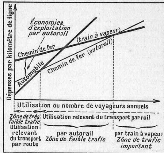
FIG. 5. — SCHÉMA INDIQUANT LES DÉPENSES D'EXPLOITATION, PAR KILOMÈTRE PARCOURU, EN FONCTION DU NOMBRE DE VOYAGEURS TRANSPORTÉS ANNUELLEMENT, POUR LES TROIS MODES DE TRANSPORT : TRAIN A VAPEUR, AUTORAIL, AUTOMOBILE
