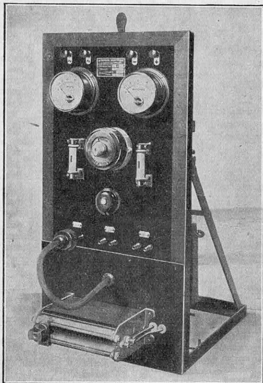
ENSEMBLE DU REDRESSEUR DE COURANT MODÈLE NORMAL « M. 10 B »
