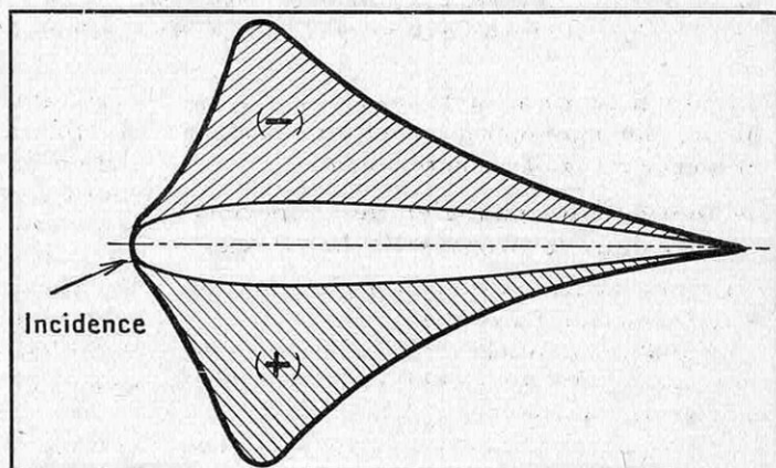
FIG. 2. — DIAGRAMMES SCHÉMATIQUES DES INTERACTIONS DE L'AIR SUR L'AILE « SYMÉTRIQUE »
