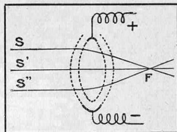
FIG. 11. — AUTRE EXPÉRIENCE MONTRANT L'ACTION D'UN CHAMP MAGNÉTIQUE SUR UN FAISCEAU CATHODIQUE
