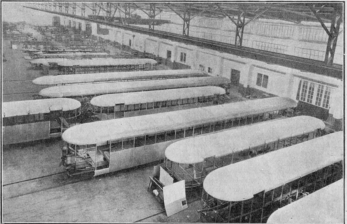
FIG. 6. — ATELIER DE FABRICATION DES « LITTORINE » (AUTORAIS FIAT), EN ITALIE
