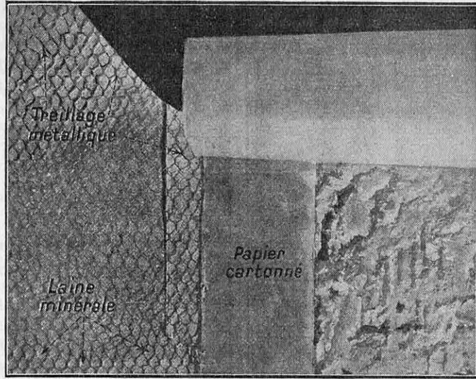
FIG. 5. — COMMENT EST RÉALISÉ, D'UNE FAÇON COMPLÈTE, L'ISOLEMENT ACOUSTIQUE D'UN STUDIO Laine minérale maintenue par treillages métalliques, papier cartonné constituent un revêtement ayant une absorption de 40 % à toutes les fréquences et assurent le silence absolu.
