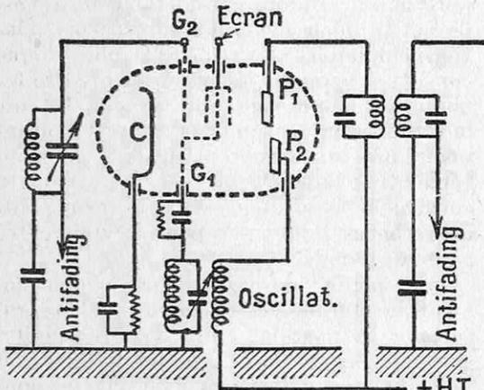
FIG. 6. — SCHEMA DE LA NOUVELLE LAMPE TRIODE-HEXODE A DEUX PLAQUES
