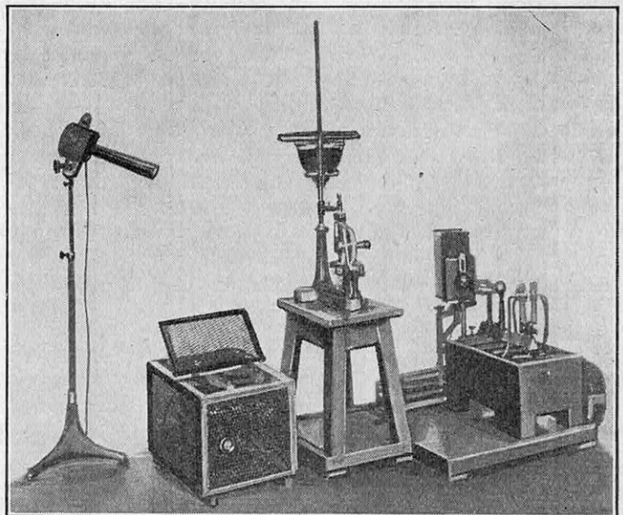
FIG. 4. — VUE D'ENSEMBLE DES APPAREILS UTILISÉS POUR LA MICROSCOPIE PAR RAYONS ULTRAVIOLETS
