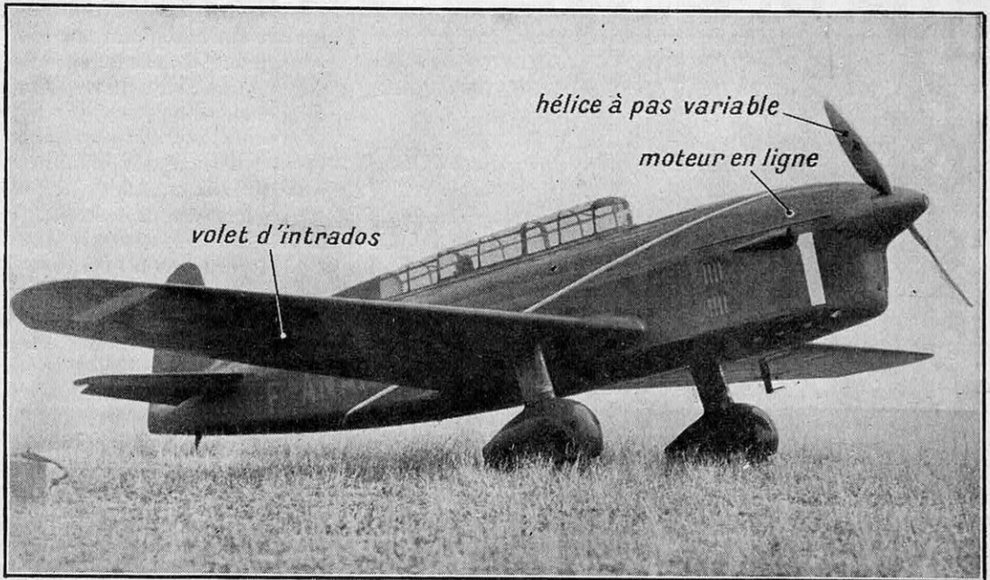
FIG. 3. — L'AVION « RAFALE » A PROFILS D'AILES « SYMÉTRIQUES »
