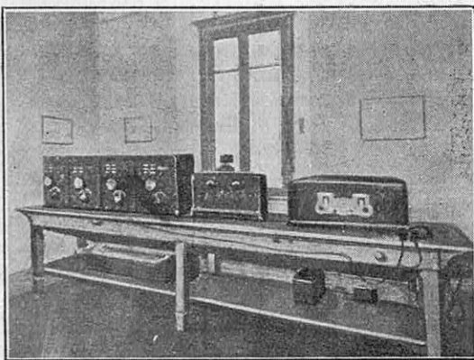
FIG. 8. — SALLE DE MESURE DES FRÉQUENCES AU CENTRE DE CONTROLE DE SESTO CALENDE
