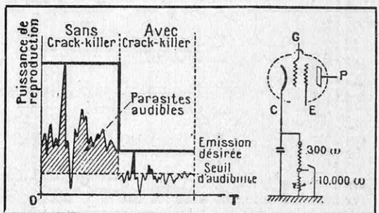
FIG. 9. — PRINCIPE DU FONCTIONNEMENT DU « CRACK-KILLER » POUR L'ÉCOUTE LOCALE
