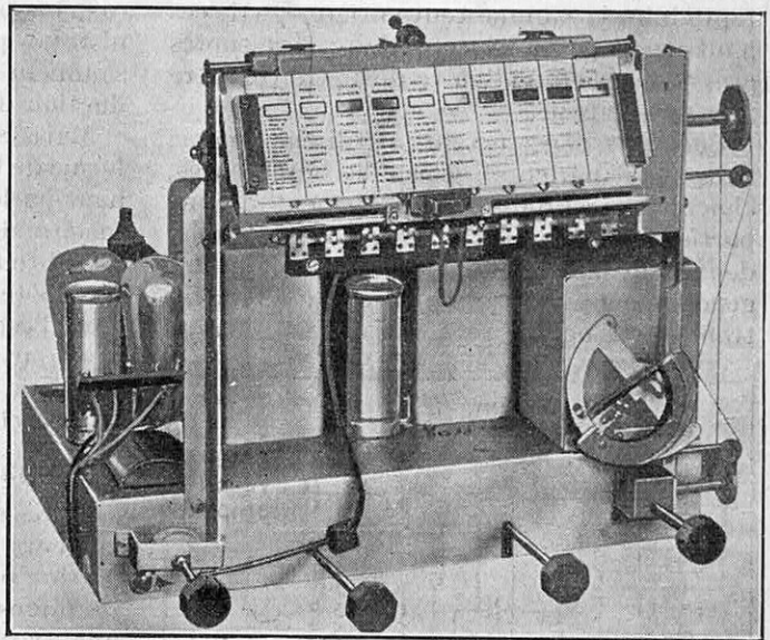
FIG. 13. — CADRAN A RÉGLAGE, DIT « NATIONAL »
