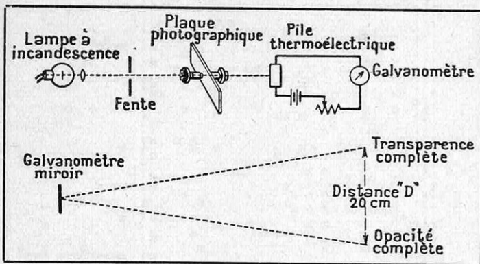
FIG. 7. — SCHÉMA DU DISPOSITIF PERMETTANT DE MESURER LA TRANSPARENCE — OU ENCORE SON INVERSE, L'OPACITÉ — D'UN CLICHÉ NÉGATIF OU POSITIF
