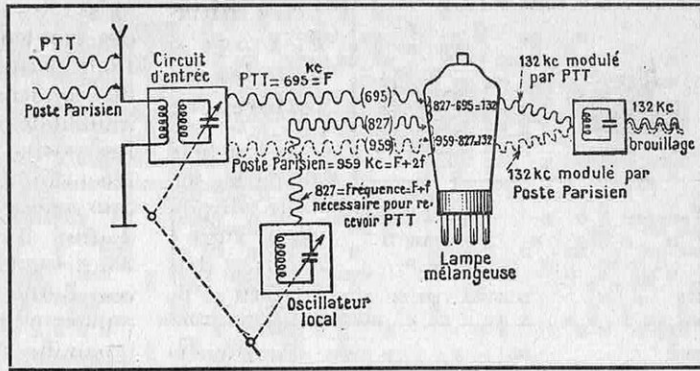
FIG. 7. — COMMENT SE PRODUIT LA « RÉCEPTION-IMAGE »
