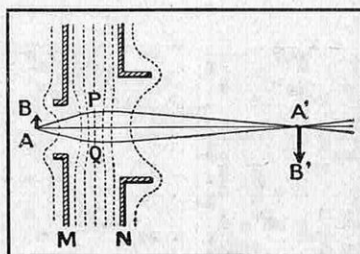
FIG. 13. — SCHEMA D'UNE LENTILLE ÉLECTRONIQUE
