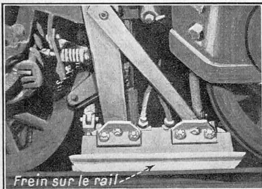
FIG. 4. — FREIN ÉLECTROMAGNÉTIQUE SUR RAIL, MONTÉ SUR UN TRAMWAY ALLEMAND, ASSURANT UN FREINAGE BEAUCOUP PLUS EFFICACE QUE LE FREINAGE SUR ROUES
