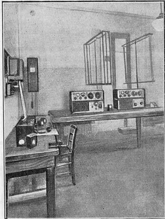
FIG. 9. — SALLE DE MESURE DU CHAMP ÉLECTROMAGNÉTIQUE A SESTO CALENDE
