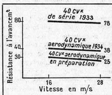
FIG. 7. — GRAPHIQUE MONTRANT LE GAIN DE LA VOITURE CI-DESSUS, EN MATIÈRE DE RÉSISTANCE A L'AVANCEMENT
