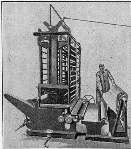
FIG. 3. — MACHINE UTILISÉE AUJOURD'HUI POUR ENDUIRE LES TISSUS DE LATEX
