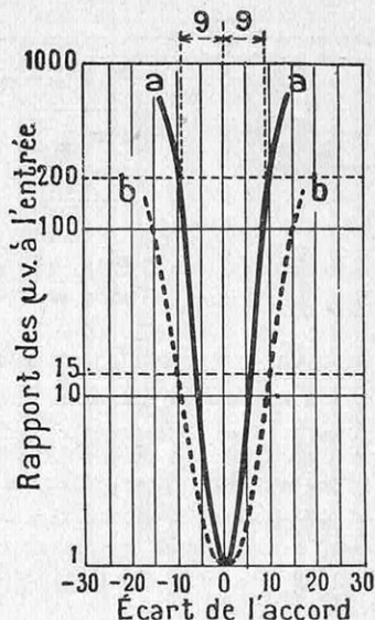
FIG. 2. — UNE GRANDE SÉLECTIVITÉ (COURBE a) DIMINUE LA BANDE DE FRÉQUENCE ET NE LAISSE PAS PASSER ÉGALEMENT TOUTES LES NOTES, COMME UNE SÉLECTIVITÉ MOINS GRANDE (COURBE b)
