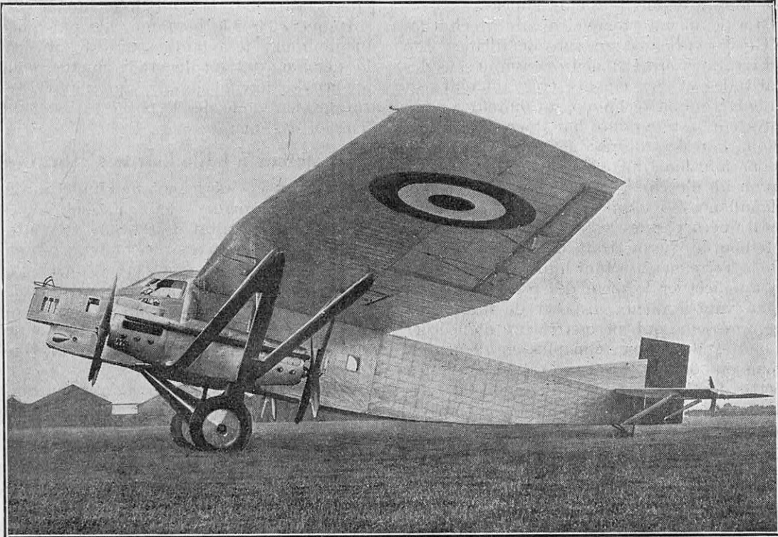
FIG. 1. — LE « FARMAN-220 » QUADRIMOTEUR EST L'UN DES PLUS PUISSANTS ET PLUS RAPIDES APPAREILS DE COMBAT ET DE BOMBARDEMENT QUI EXISTENT A L'HEURE ACTUELLE. IL PEUT TRANSPORTER 5.000 KILOGRAMMES SUR 1.000 KILOMÈTRES DE DISTANCE ET ATTEINT UNE VITESSE DE 300 KILOMÈTRES A L'HEURE A 4.000 MÈTRES D'ALTITUDE
