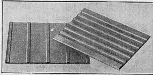
FIG. 4. — PLANCHER ANTIVIBRATOIRE SERVANT DE SUPPORT A UNE MACHINE-OUTIL Ce plancher, très spécial, est fabriqué avec du Revertex, c'est-à-dire du latex concentré contenant jusqu'à 75 % de caoutchouc.
