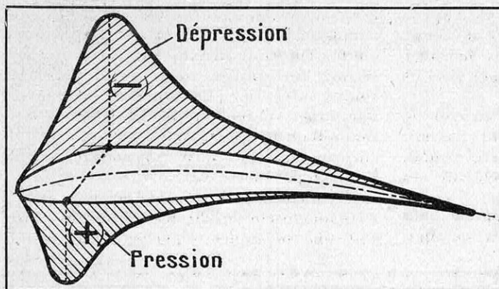
FIG. 1. — DIAGRAMMES SCHÉMATIQUES DES INTERACTIONS DE L'AIR SUR L'AILE D'AVION CLASSIQUE
