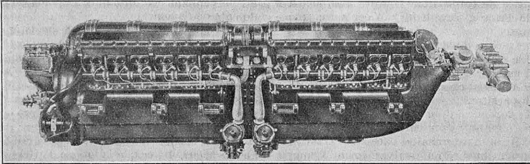
FIG. 4. — VOICI LE DOUBLE MOTEUR « FIAT » QUI ÉQUIPE L'HYDRAVION ITALIEN « MACCHI », SUR LEQUEL LE PILOTE ITALIEN AGELLO A BATTU RÉCEMMENT TOUS LES RECORDS DU MONDE DE VITESSE EN ATTEIGNANT 709 KILOMÈTRES A L'HEURE
