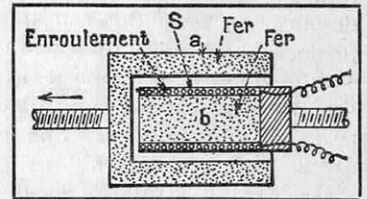
FIG. 5. — SELF VARIABLE A NOYAU DE FER DOUX
