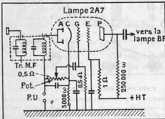
FIG. 14. — EMPLOI D'UN POTENTIOMÈTRE RÉGULATEUR DE L'INTENSITÉ SONORE
