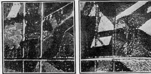
FIG. 15. — PHOTOGRAPHIES D'UNE MÊME CATHODE OBTENUES : CELLE DE GAUCHE, AVEC UN MICROSCOPE OPTIQUE ; CELLE DE DROITE, AVEC LE MICROSCOPE ÉLECTRONIQUE
