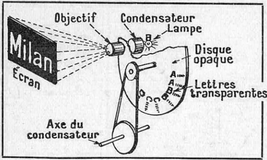
FIG. 8. — DISPOSITIF FAISANT APPARAÎTRE LES NOMS LUMINEUX DES STATIONS SUR LESQUELLES LE POSTE EST ACCORDÉ
