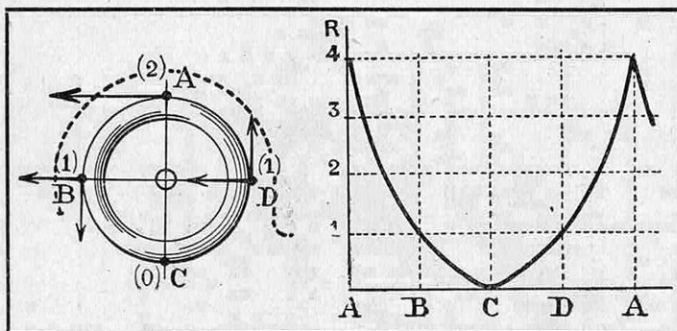
FIG. 9. — LA RÉPARTITION DES RÉSISTANCES AÉRODYNAMIQUES D'UNE ROUE QUI AVANCE SUR LA ROUTE. Au point C (contact avec le sol), la vitesse, relativement à l'air, est nulle. En B et en D, elle est égale à la vitesse de translation de la voiture. En A, elle est double de cette translation. Le graphique adjoint au schéma de la roue en mouvement montre comment varie la résistance aérodynamique sur les divers points de la roue, en vertu du schéma de gauche. Cette résistance croît immensément au-dessus du diamètre B D. C'est pourquoi l'aile doit masquer toute la moitié supérieure de la roue.
