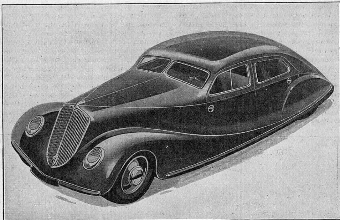
FIG. 6. — AUTRE RÉALISATION (« RENAULT ») TENDANT A SE RAPPROCHER DU PROFIL AÉRODYNAMIQUE THÉORIQUE TOUT EN COMPOSANT AVEC LES FORMES ACTUELLES DE L'AUTO
