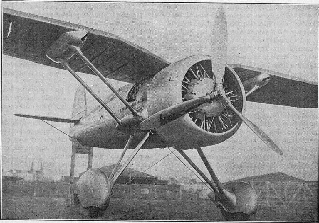
FIG. 3. — VOICI L'UNE DES CURIOSITÉS DU SALON : L'AVION DE CHASSE POLONAIS « P. Z. L. », ARMÉ DE DEUX CANONS AUTOMATIQUES OERLIKON. CET APPAREIL A DES QUALITÉS DE VITESSE ET DE PUISSANCE ASCENSIONNELLES TOUT A FAIT REMARQUABLES
