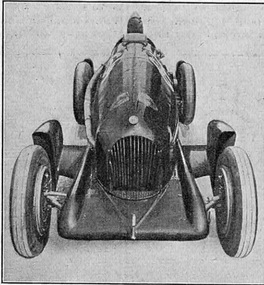
FIG. 10. — UNE VOITURE DE COURSE DE CARROSSERIE ORIGINALE, MAIS PRATIQUEMENT EFFICACE POUR LES GRANDES VITESSES. Dans cette forme, le constructeur a sacrifié la résistance avant des roues (et son accroissement par effet Magnus); mais il a fait suivre les roues d'un fuselage destiné à annuler leurs tourbillons de traînée. Par contre, le radiateur est réduit, parce que l'air qui s'y engouffre est « guidé » par le plateau avant; celui-ci, d'autre part, guide les filets de l'air inséré entre le sol et la voiture.
