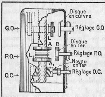
FIG. 4. — ENSEMBLE D'ACCORD POUR TOUTES ONDES. LES ENROULEMENTS P. O. ET O. C. (ONDES COURTES) SONT BOBINÉS SUR NOYAUX DE FER
