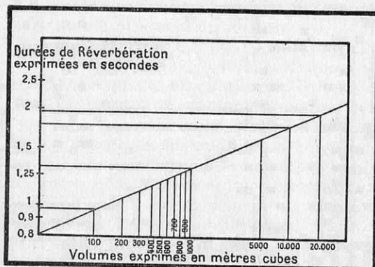
FIG. 2. — LA « RÉVERBÉRATION » DOIT ÊTRE ÉTUDIÉE SELON LE VOLUME DE LA SALLE Ce diagramme, établi empiriquement par F.-R. Watson, professeur de physique expérimentale à l'Université de l'Illinois (Etats-Unis), donne les durées les plus convenables de la réverbération en fonction du volume de la salle.
