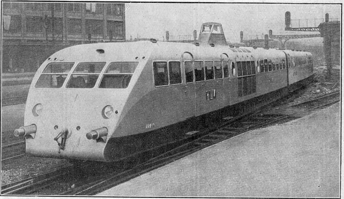
FIG. 1. - L'AUTORAIL P.-L.-M. «BUGATTI» QUI A ASSURÉ L'ÉTÉ DERNIER LE SERVICE PARIS-VICHY, ET QUI ASSURE, DEPUIS LE MOIS DE NOVEMBRE 1934, LE SERVICE PARIS-LYON
