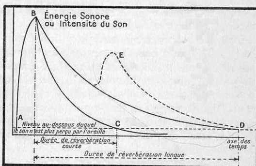
FIG. 3. — DÉCROISSANCE DU SON EN FONCTION DES DURÉES DE RÉVERBÉRATION Si la réverbération est irrégulière (courbe ED), et si le temps s'écoulant entre B et E dépasse 1/12 e de seconde, l'auditeur a la sensation désagréable de la répétition du son, d'un écho.
