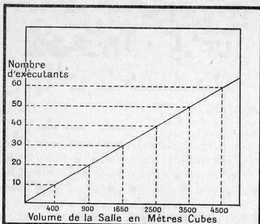
FIG. 1. — LE VOLUME D'UNE SALLE DOIT VARIER AVEC LE NOMBRE D'EXÉCUTANTS Diagramme montrant le volume le plus convenable pour une salle d'émission en fonction du nombre d'exécutants qui doivent y prendre place.
