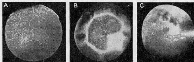
FIG. 16. — TROIS PHOTOGRAPHIES DE CATHODES OBTENUES AU MOYEN DU MICROSCOPE ÉLECTRONIQUE
