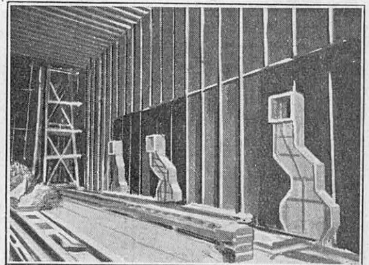
FIG. 7. — LES CONDUITS D'AÉRATION SONT ÉTUDIÉS TOUT SPÉCIALEMENT POUR ÉVITER LE PASSAGE DES ONDES SONORES
