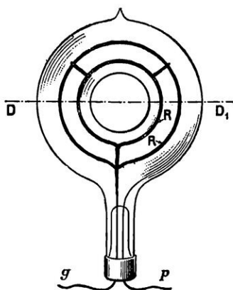
FIG. 2. — ASPECT EXTÉRIEUR DE LA CELLULE DE SCHRÖTER
