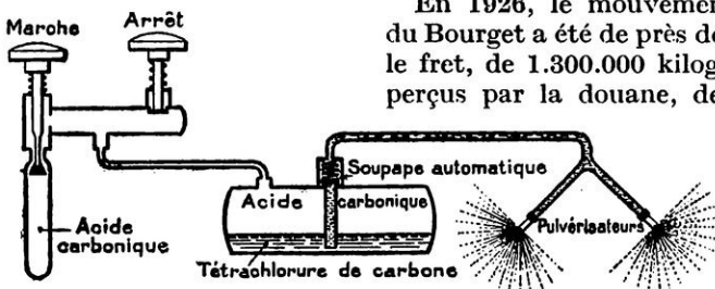
SCHÉMA DE FONCTIONNEMENT D'UN EXTINCTEUR D'INCENDIE AU TÉTRACHLORURE DE CARBONE
