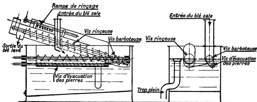
FIG. 5. — SCHÉMA DE LA MACHINE À LÁVER LE BLÉ
