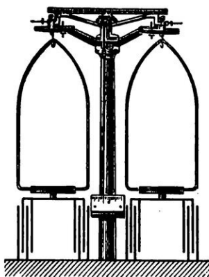
FIG. 7. — BALANCE A AMORTISSEURS
