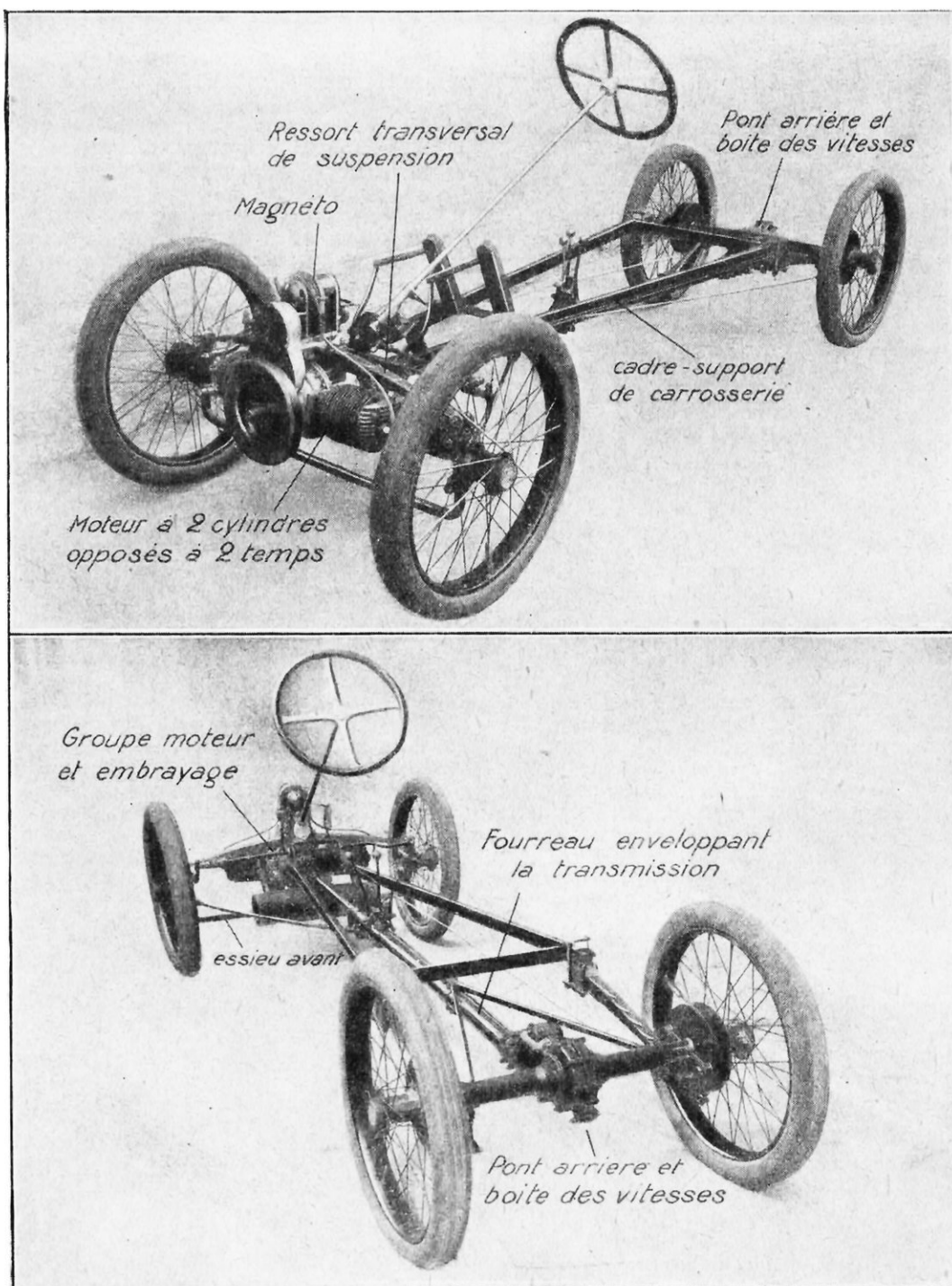
FIG. 3. — LES MÉCANISMES DE LA VOITURE SIMA-VIOLET
