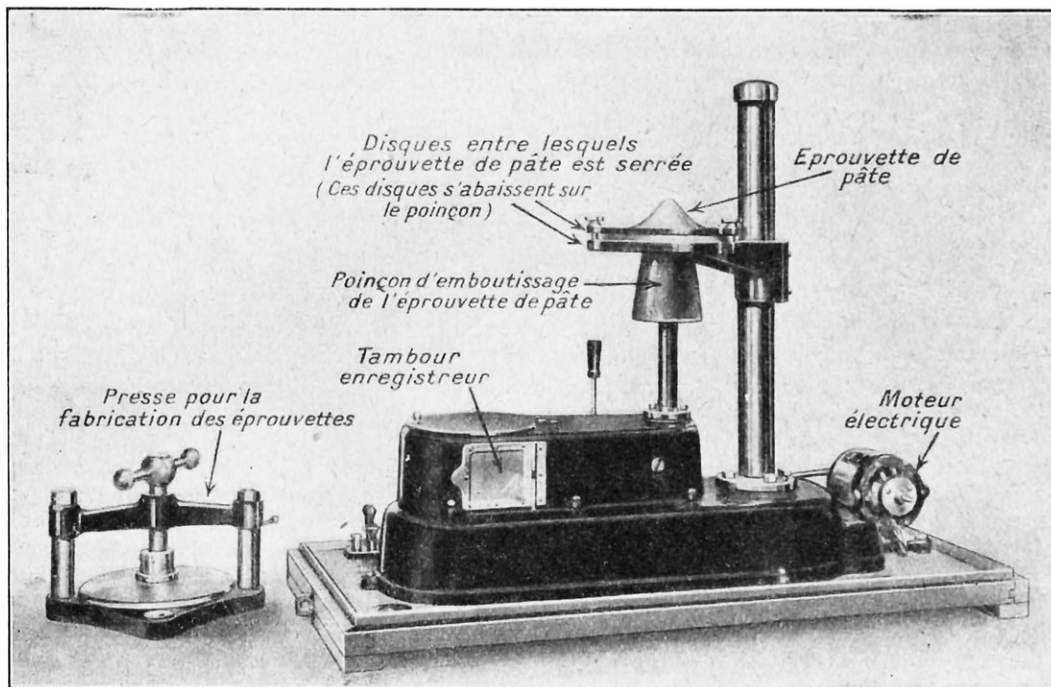
FIG. 12. — APPAREIL PERMETTANT DE SE RENDRE COMPTE DE LA VALEUR BOULANGÈRE D'UNE FARINE
