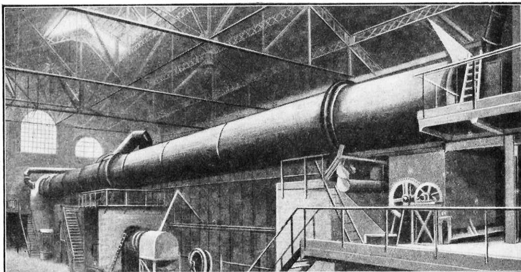
L'ALUMINE HYDRATÉE, PROVENANT DU TRAITEMENT DE LA BAUXITE, MINÉRAI DE L'ALUMINIUM, EST CALCINÉE A 1.200 DEGRÉS DANS CE LONG FOUR CYLINDRIQUE
