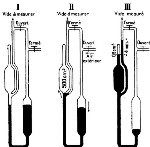
FIG. 2. - COMMENT ON MESURE UN VIDE ÉLEVÉ
