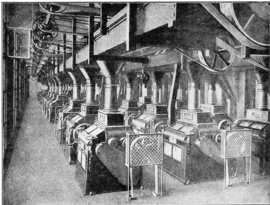
FIG. 8. — VUE D'ENSEMBLE D'UNE SALLE DE MOULINS A CYLINDRES POUR LA MOUTURE DU BLÉ
