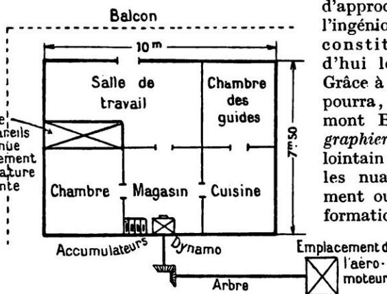
PLAN DE L'OBSERVATOIRE VALLOT Disposition de l'organisation projetée par M. Dina.
