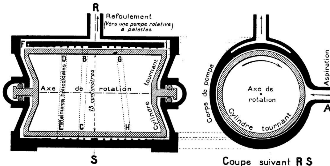
FIG. 10. — UNE DES DERNIÈRES POMPES MOLÉCULAIRES
