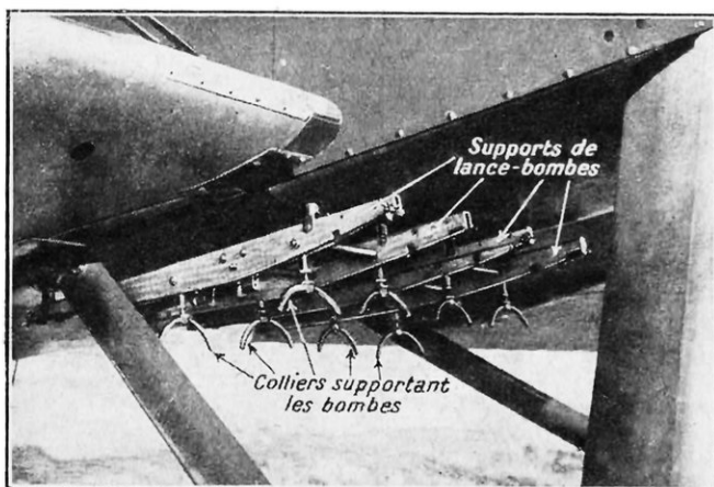
INSTALLATION D'UN LANCE-BOMBES SUR AVION POTEZ 25
