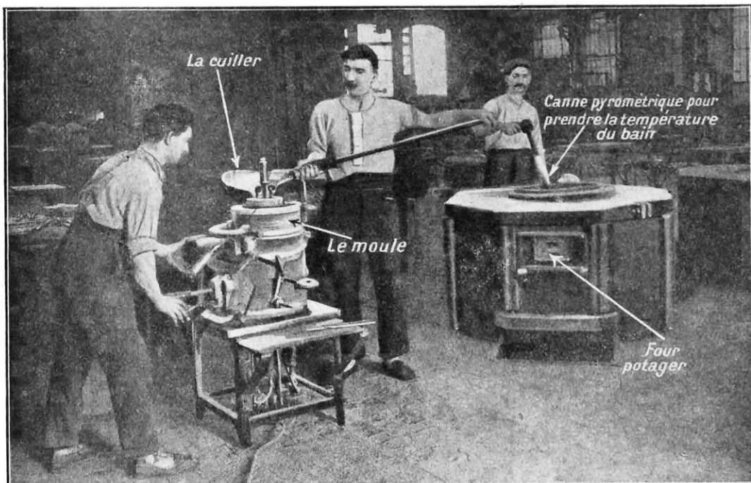
LES ALLIAGES D'ALUMINIUM, DITS « ALLIAGES LÉGERS », SONT TRÈS EMPLOYÉS. ON VOIT ICI LA COUÉE EN COQUILLE D'UNE PIÈCE D'AUTOMOBILE
