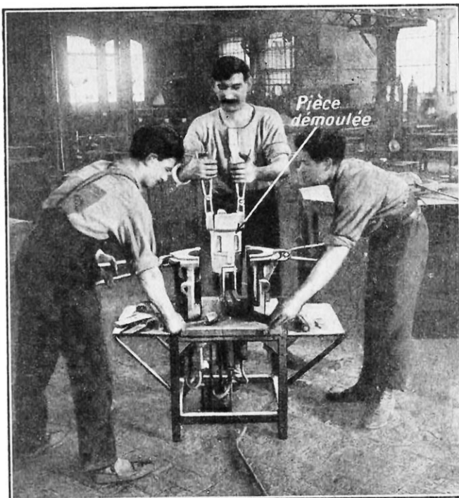
LE MOULE SE SÉPARE EN DEUX PARTIES POUR PERMETTRE D'EN RETIRER AISÉMENT LA PIÈCE COULÉE, APRÈS REFROIDISSEMENT
