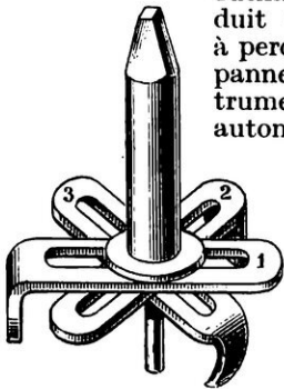
CET OUTIL PERMET DE PERCER FACILEMENT DES TROUS DANS LE MÉTAL, L'ÉBONITE, ETC.
