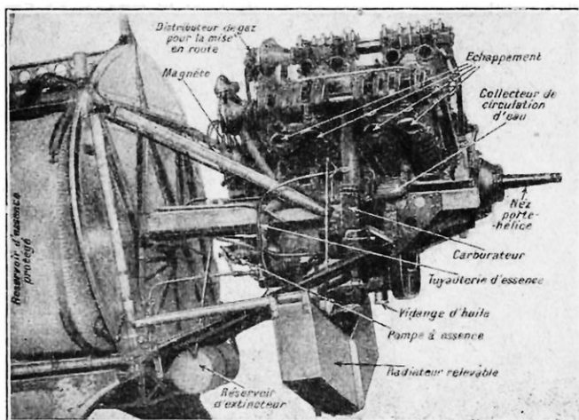
MOTEUR LORRAINE-DIETRICH 450 C. V. SUR BRÉGUET 19 C'est le moteur à 12 cylindres qui, suralimenté par un turbo-compresseur Raleau, a permis à Calizzo d'atteindre 12.400 mètres d'altitude.
