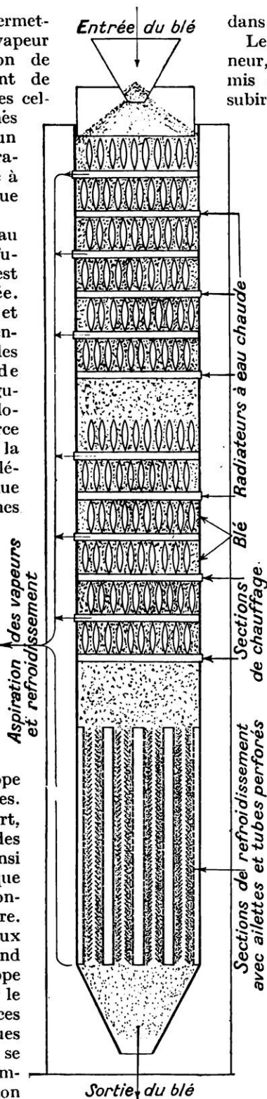
FIG. 7. COUPE D'UN CONDITION- NEUR POUR LE BLÉ
