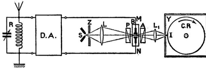
FIG. 5. — RÉCEPTEUR UTILISANT LA CELLULE KAROLUS
