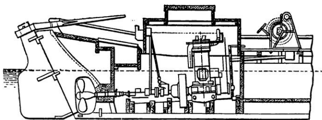
FIG. 1. — SCHÉMA D'INSTALLATION D'UN MOTEUR A BORD D'UN BATEAU DE PÊCHE
