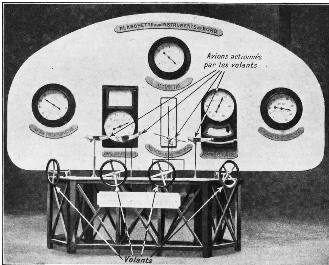
UN TABLEAU PARTICULIÈREMENT SUGGESTIF DES APPAREILS DE BORD D'UN AVION Les visiteurs du Salon pouvaient, en actionnant les volants, faire prendre aux avions-maquettes des déplacements qui étaient traduits immédiatement sur les appareils que le pilote a constamment sous les yeux.
