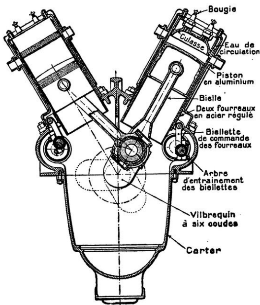
COUPE TRANSVERSALE DU MOTEUR PANHARD-LEVASSOR SANS SOUPAPE
