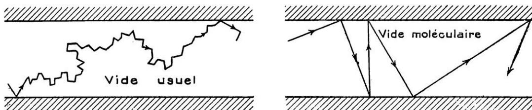
FIG. 9. — LES DEUX SORTES DE VIDES
