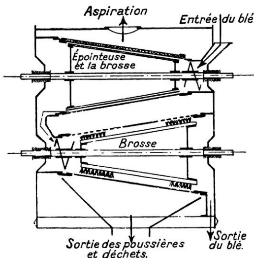
FIG. 2. — MACHINE COMBINÉE, ÉPOINTEUSE ET BROSE, POUR LE NETTOYAGE DU BLÉ
