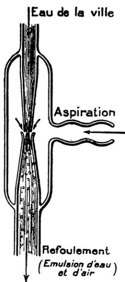
FIG. 5. — TROMPE À EAU
