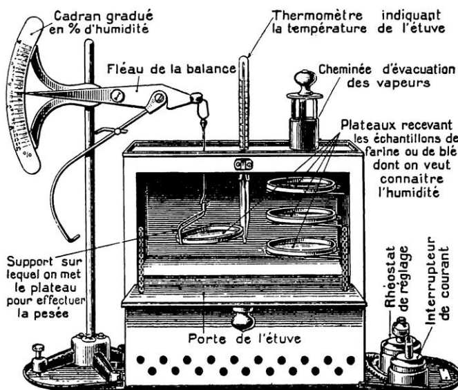
FIG. 11. — BALANCE-ÉTUVE PERMETTANT DE LIRE DIRECTEMENT L'HUMIDITÉ DU BLÉ
