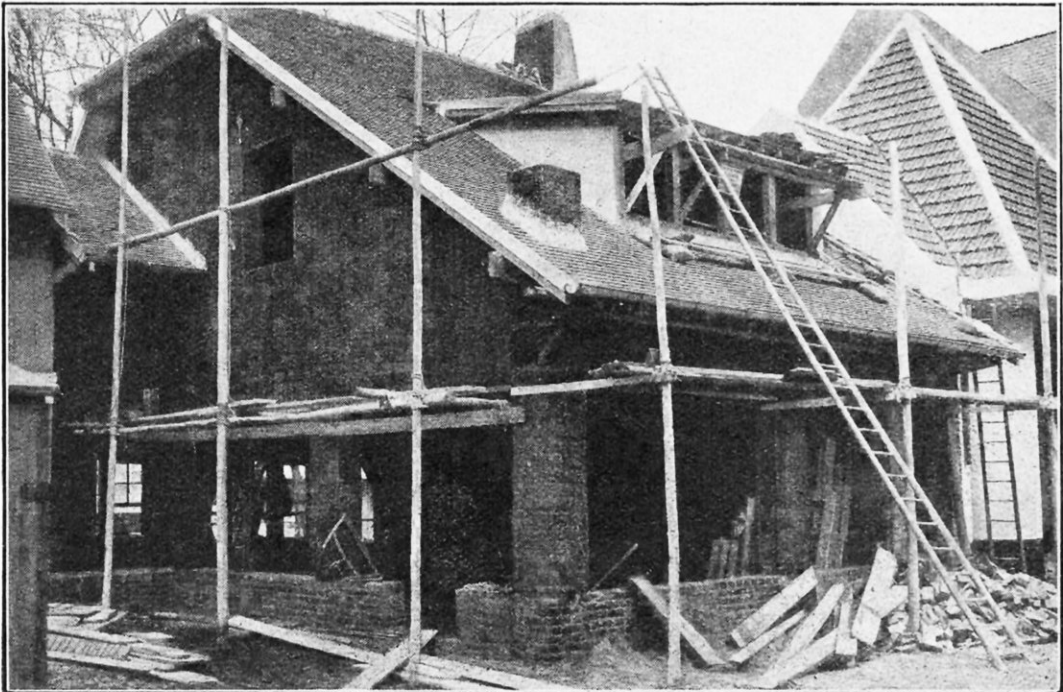
LES MURS ET LES CLOISONS DE L'AUBERGE DU VILLAGE FRANÇAIS, A L'EXPOSITION DES ARTS DÉCORATIFS, ONT ÉTÉ CONFECTIONNÉS AVEC CES PANNEAUX DE PAILLE COMPRIMÉE
