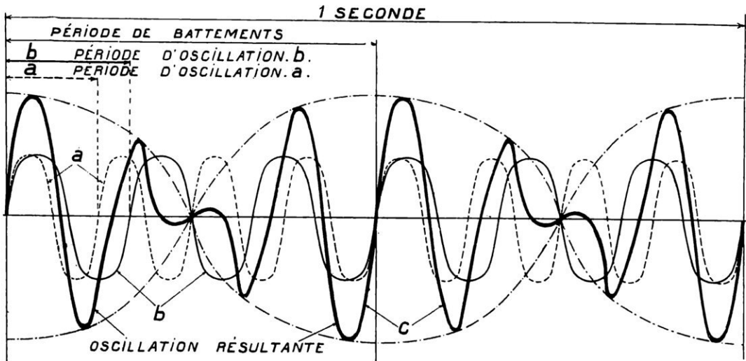
FIG. 1. — COURBES PERMETTANT D'EXPLIQUER LE PRINCIPE DU MONTAGE SUPERHÉTÉRODYNE
