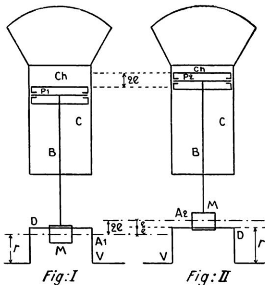
SCHÉMA DE PRINCIPE DE L'APPAREIL (Voir dans le texte l'explication des lettres)
