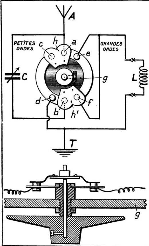
FIG. 2. — COMMUTATEUR SÉRIE-PARALLÈLE MANGÉVRE PAR UN BOUTON
