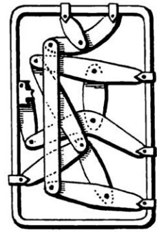
FIG. 2 VUE DU MÉCANISME MONTRANT LES DIFFÉRENTES BIELLETES QUI LE CONSTITUENT
