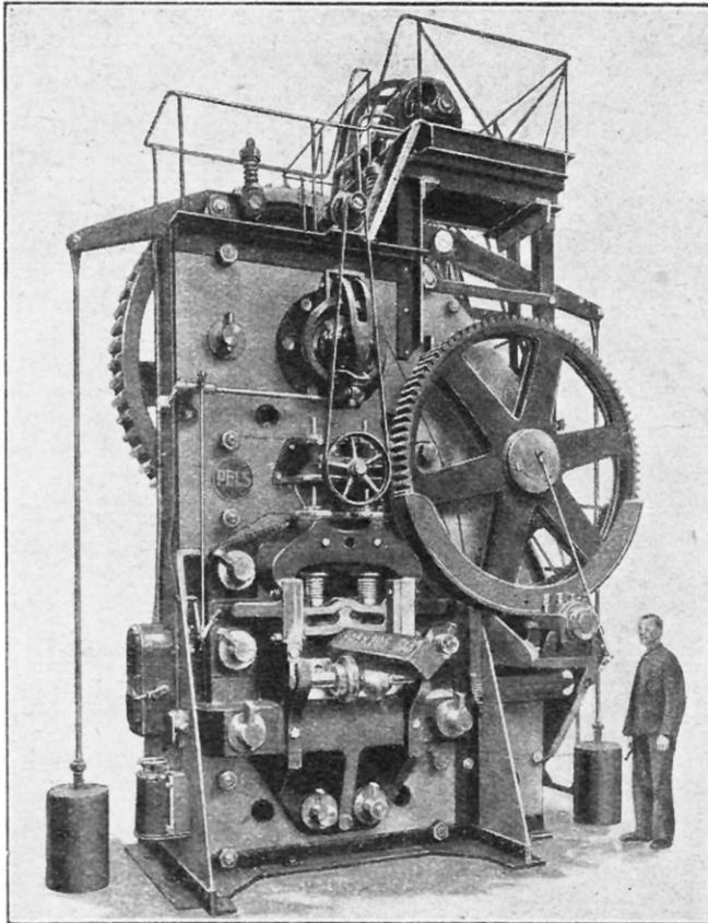
LA PLUS GRANDE CISAILLE A ENGRENAGES DU MONDE On aperçoit la barre d'acier de 20 x 20 cm. que la machine est en train de tronçonner. La pression totale réalisée par la cisaille est de 1.500 tonnes. L'énorme machine est actionnée par un moteur de 100 CV., visible sur la plate-forme supérieure
