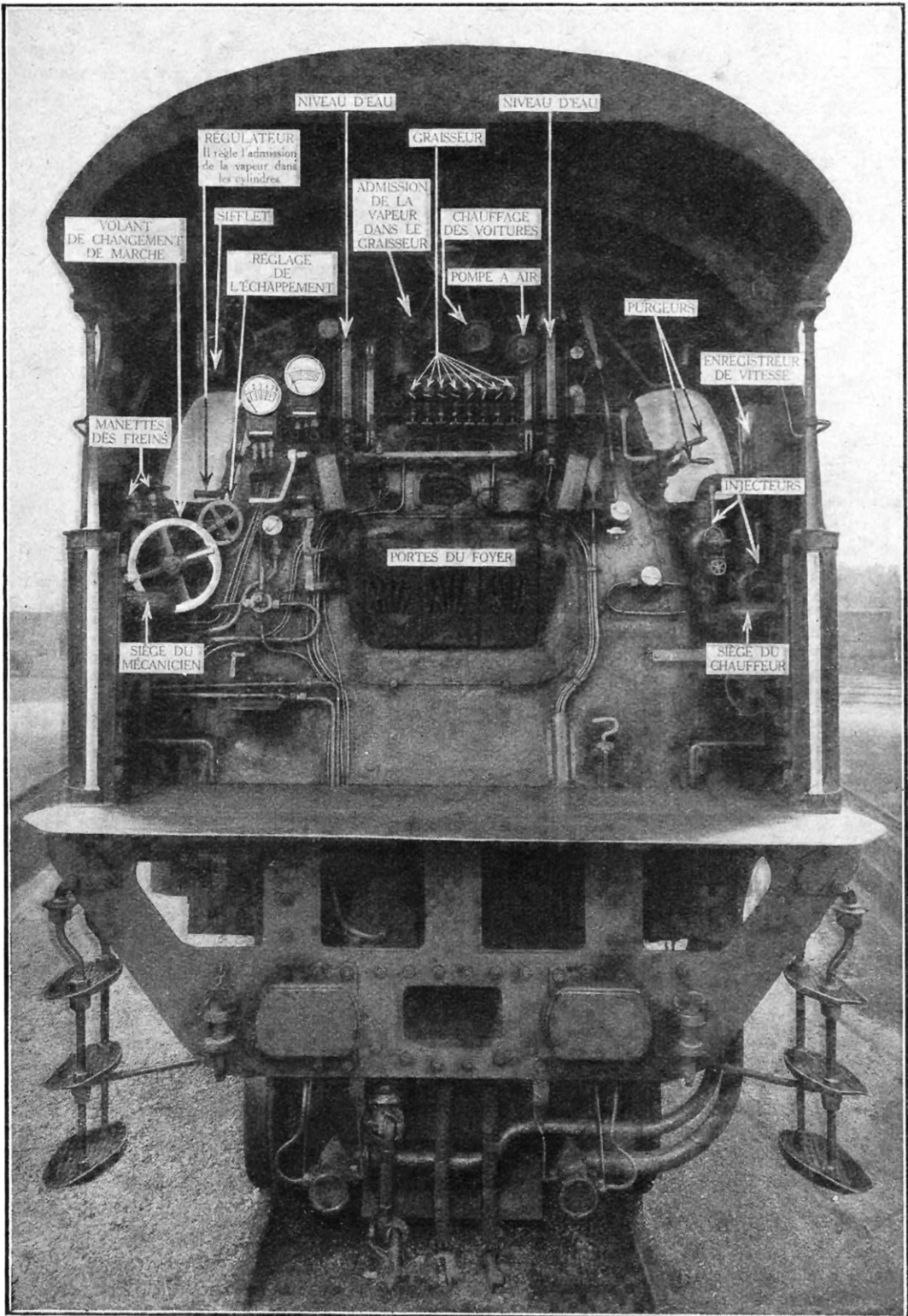
LES PRINCIPAUX ORGANES DE MANŒUVRE ET DE CONTRÔLE QUE LE MÉCANICIEN ET LE CHAUFFEUR D'UNE LOCOMOTIVE DOIVENT ACTIONNER ET CONSULTER DANS LEUR ABRU
