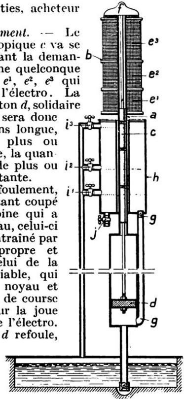
FIG. 3. — SCHEMA DE L'APPAREIL A DOUBLE CONTROLE POUR LA DISTRIBUTION DES ESSENCES DANS LES GARAGES
