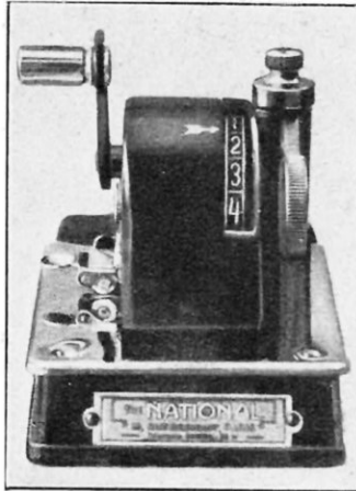
MACHINE A CHÈQUES, MODÈLE « PERSONNEL »
