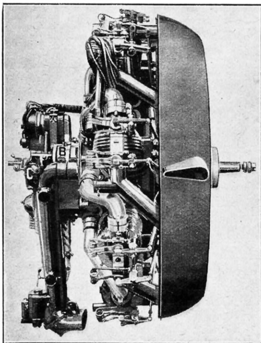
VUE DE PROFIL DU MOTEUR MUNI DU DISPOSITIF DAMBLANC
