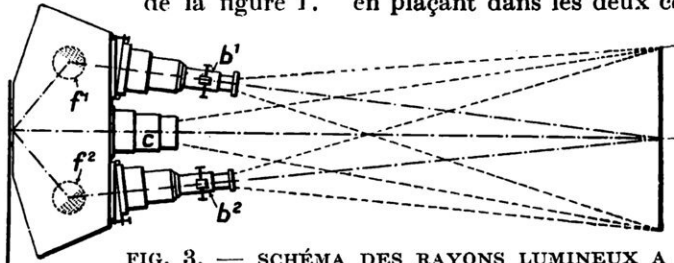
FIG. 3. — SCHÉMA DES RAYONS LUMINEUX A L'INTÉRIEUR ET A L'EXTÉRIEUR DE LA LANTERNE, LORSQUE CELLE-CI EST DISPOSÉE POUR LA PROJECTION DES VUES OPAQUES (CARTES POSTALES, ETC.)
