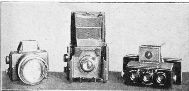
A GAUCHE, APPAREIL MUNI D'UN OBJECTIF DE GRANDE OUVERTURE POUR LA PRISE DES VUES PEU ÉCLAIRÉES ; AU CENTRE, UN APPAREIL COURANT ; A DROITE, UNE JUMELLE STÉRÉOSCOPIQUE POURVUE D'UN OBJECTIF CENTRAL SERVANT DE VISEUR
