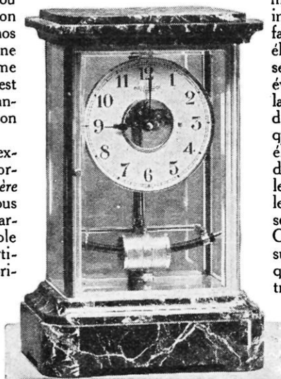
Un des nombreux modèles de la « Bulle-Clock »
