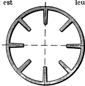
FIG. 7. — TUBE A FUMÉE MUNI D'AILLETTES
