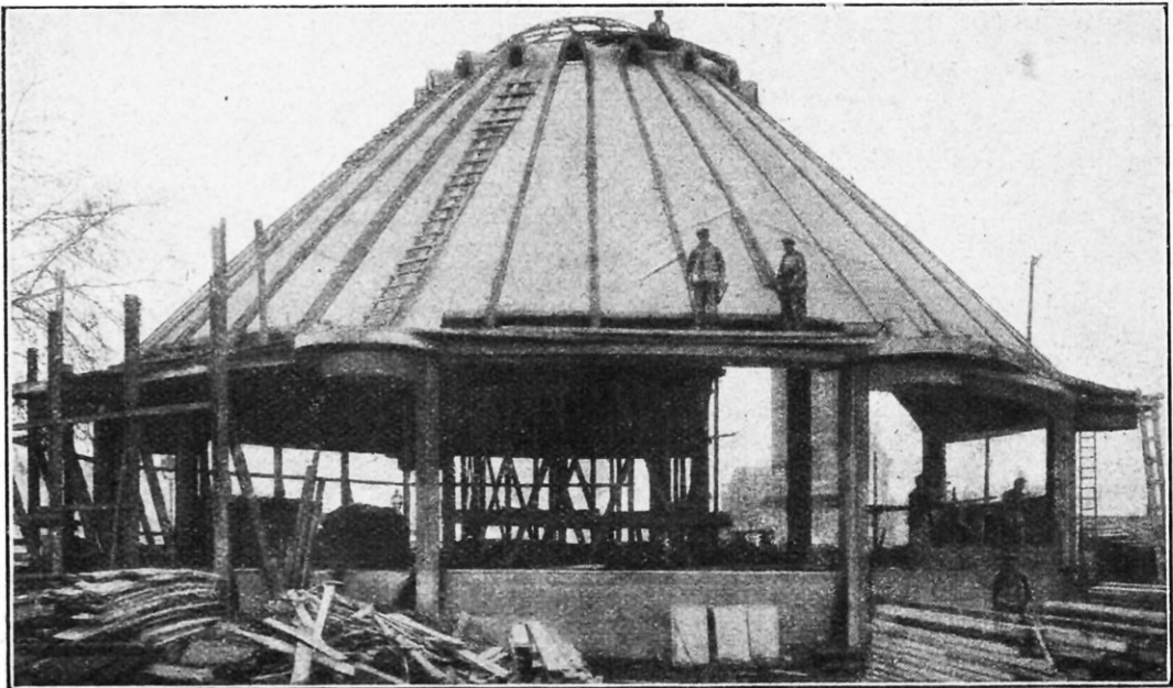
POUR LA TOITURE DU PAVILLON PRIMAVERA, A L'EXPOSITION DES ARTS DÉCORATIFS, LE SOLOMITE A ÉTÉ UTILISÉ COMME COFFRAGE ET ISOLANT THERMIQUE
