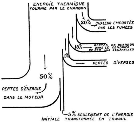
FIG. 9. — SCHEMA MONTRANT LES PERTES QUE LA TRANSFORMATION, SUR LES LOCOMOTIVES, DE L'ÉNERGIE CALORIFIQUE DU CHARBON EN TRAVAIL MÉCANIQUE ENTRAÎNE
