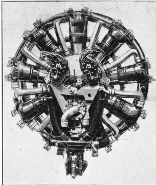
L'APPAREIL DAMBLANC MONTÉ SUR UN MOTEUR D'AVIATION (SALMONSON 300 CV)
